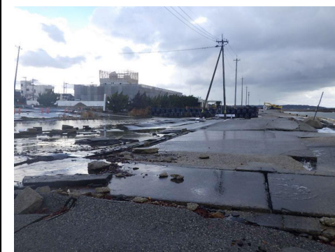
臨港道路周辺の破損状況
