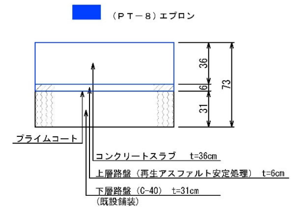
舗装構成図
