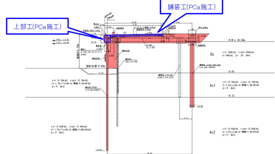
標準断面図
