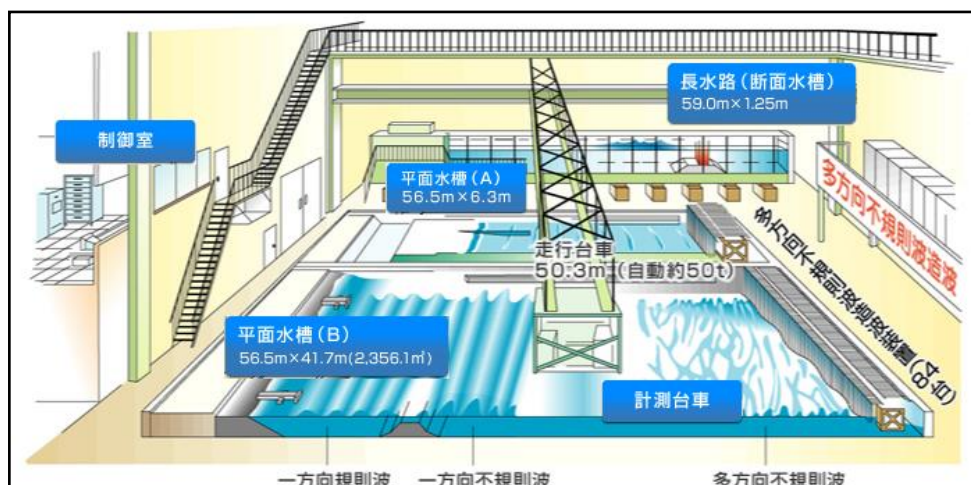
水理実験場 設備 イメージ図
